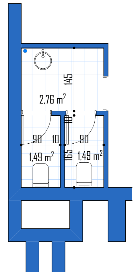
TOILETTES LOCAL POMPEIER
